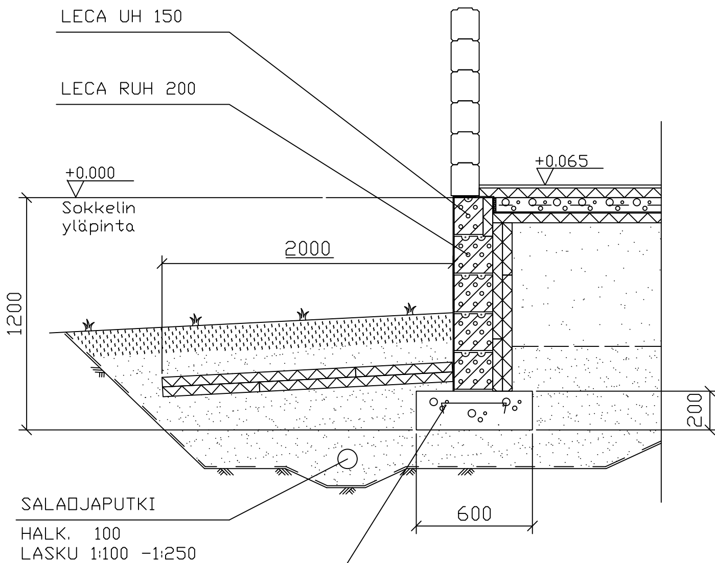
Perustusleikkaus (1:20)
