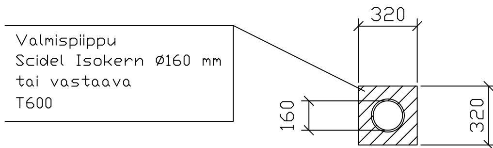
Hormileikkaus (1:20)
