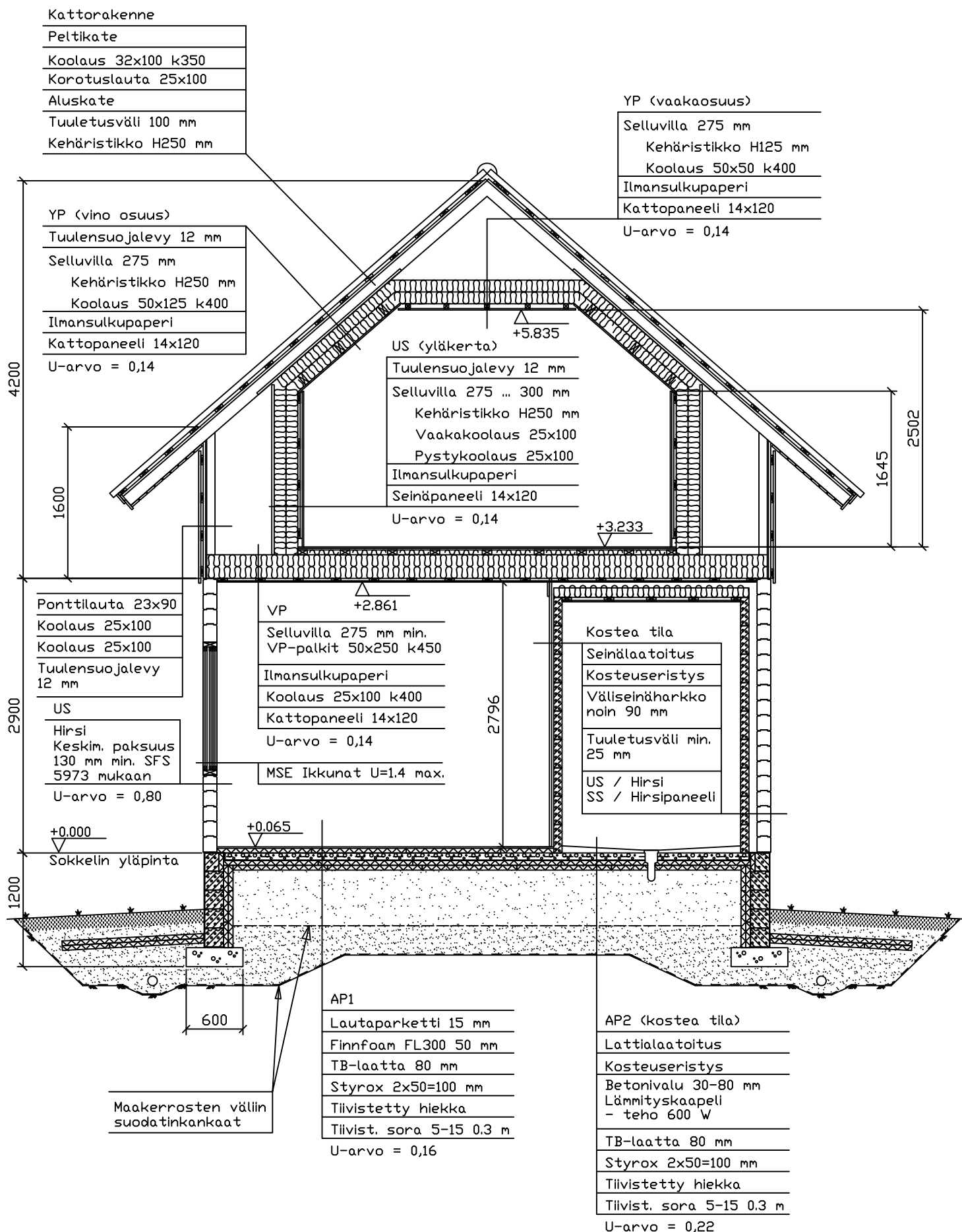
Leikkaus A-A (1:50)
